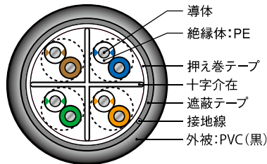
【断面構造図】
